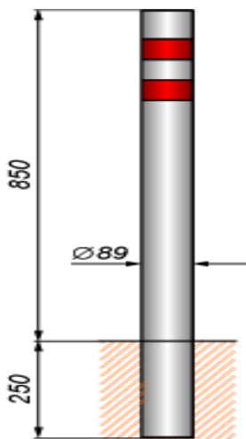
Рис. 4. Внешний вид и размеры столбика ограждения
